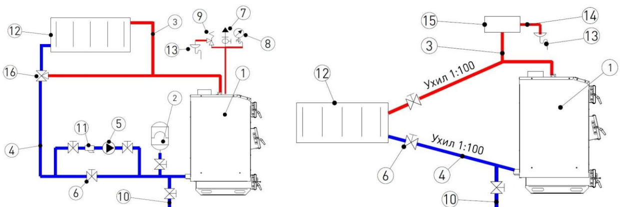
Рисунок 4 – Схеми підключення котла до системи опалення
